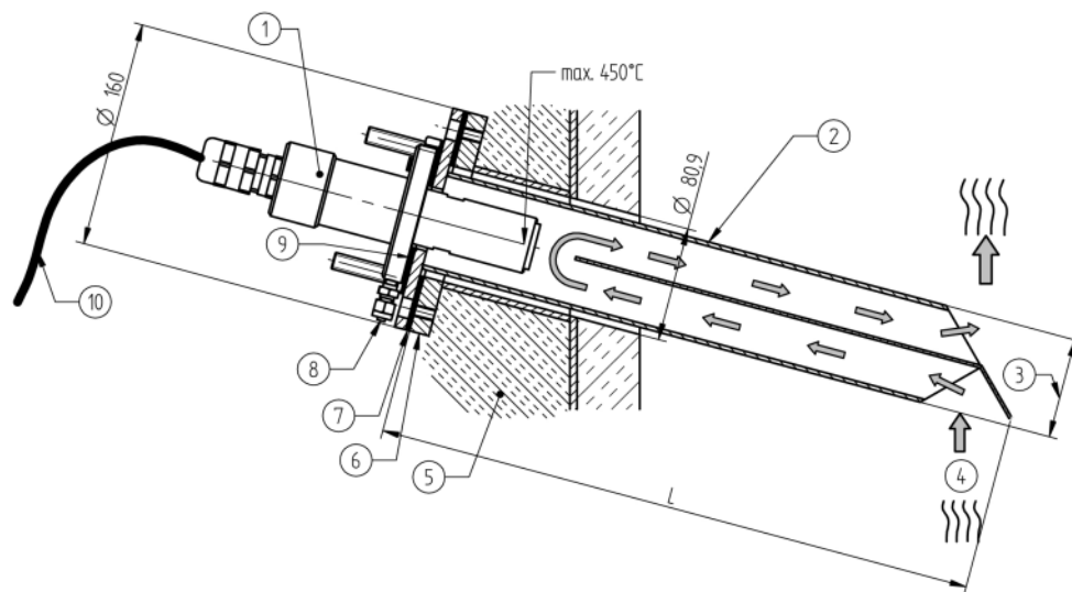
Fig. 1-2 Plan coté sonde KS1D-Ex avec tube de renvoi des gaz d'échappement
