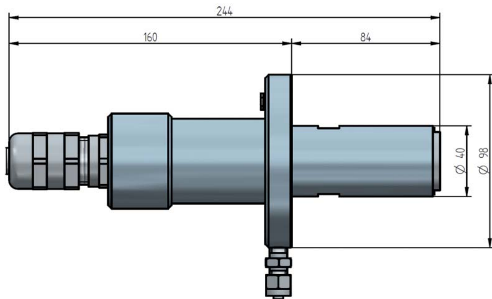
Fig. 1-1 Sonde Combinée KS1D-Ex (ZPF2)
