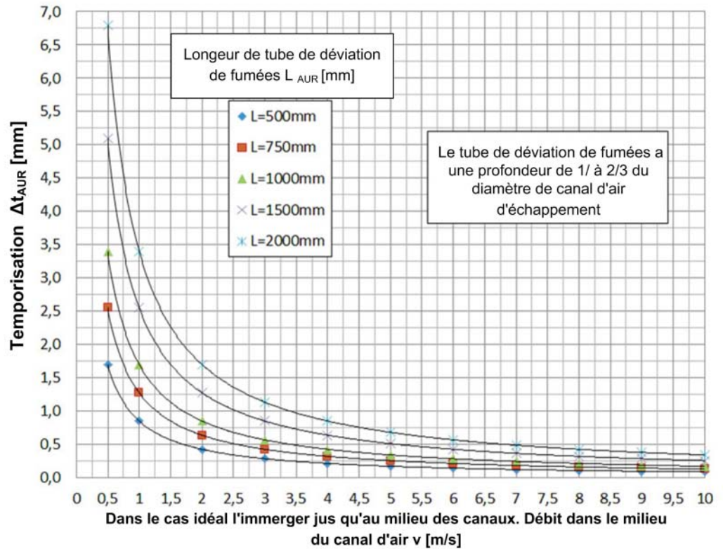
Fig. 1-4 Tube de déviation de fumées -Temporisation en fonction de la vitesse dans le canal d'air dépendent aux différentes longueurs de tube de déviation de fumées
