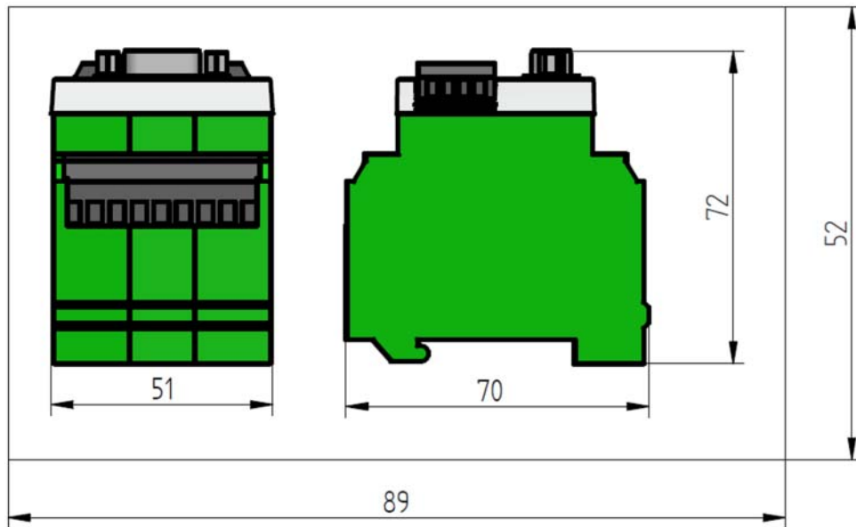
Fig. 1-1 Abmessungen PBM100
