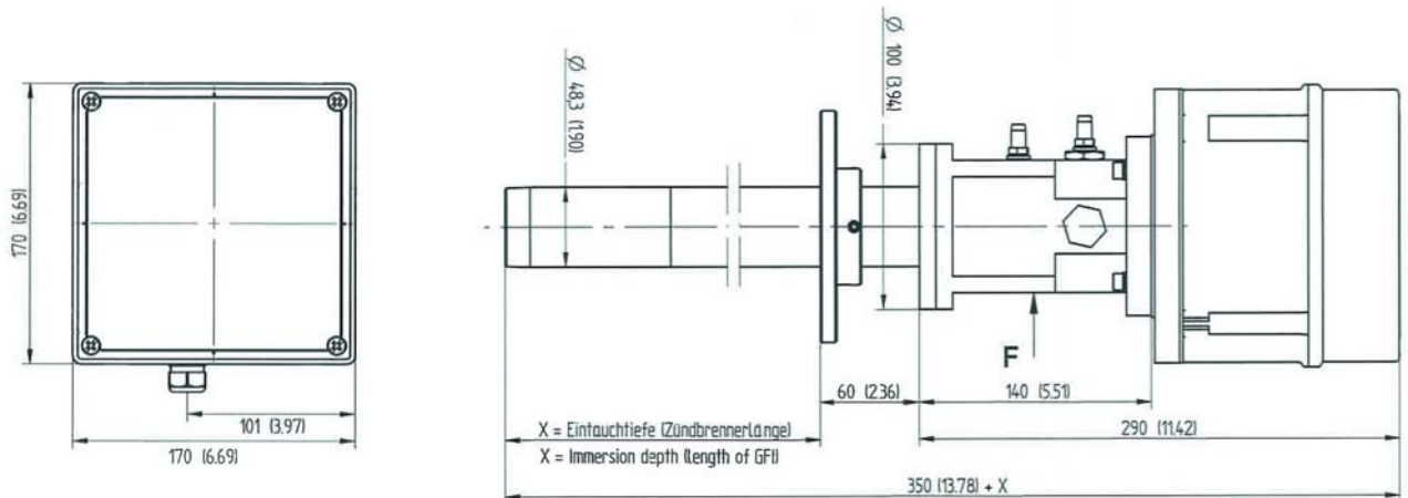
Fig. 4 Abmessungen GFI48 Zündbrenner Ex-Zone II
