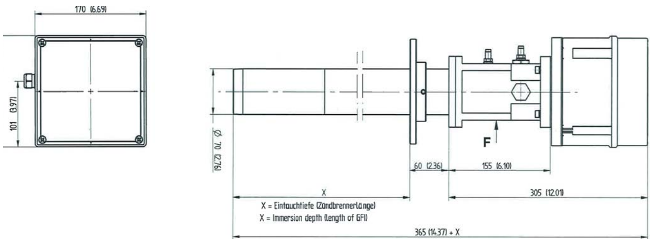
Fig. 4 Abmessungen GFI70 Zündbrenner Ex-Zone II
