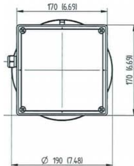
Fig. 10 Abmessungen Integrierte Leistungseinheit Ex-Zone II
