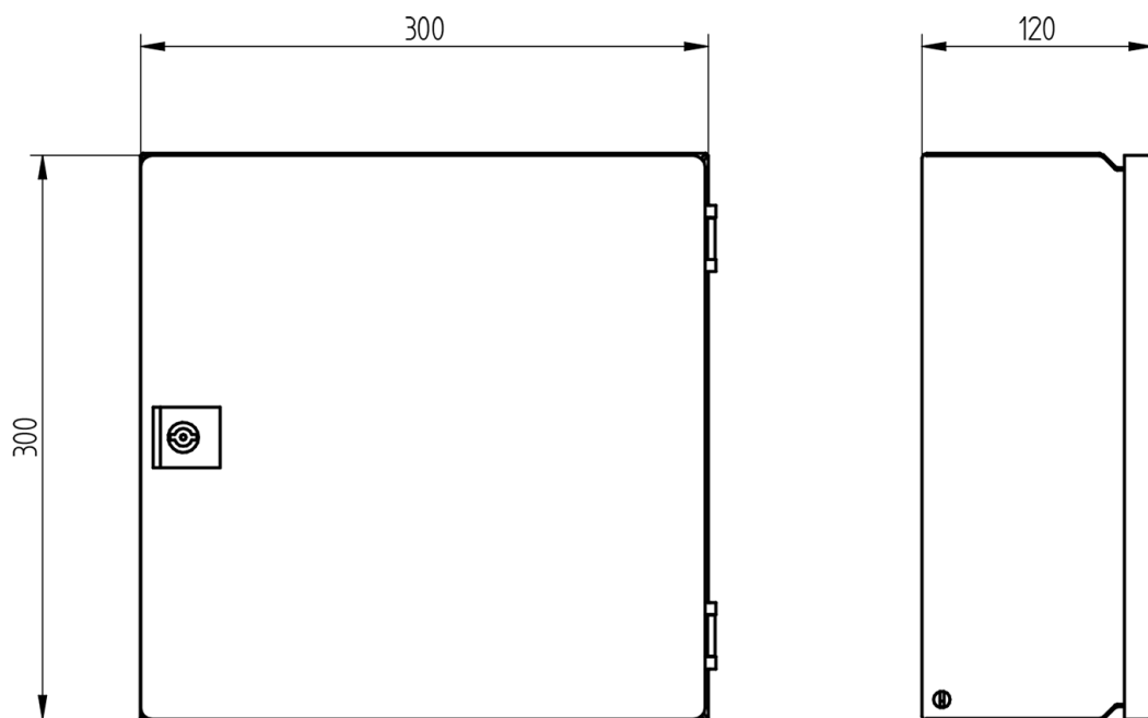
Fig. 1 Externes Stahlgehäuse für Wandmontage „Hochenergiezünder HEI600“
