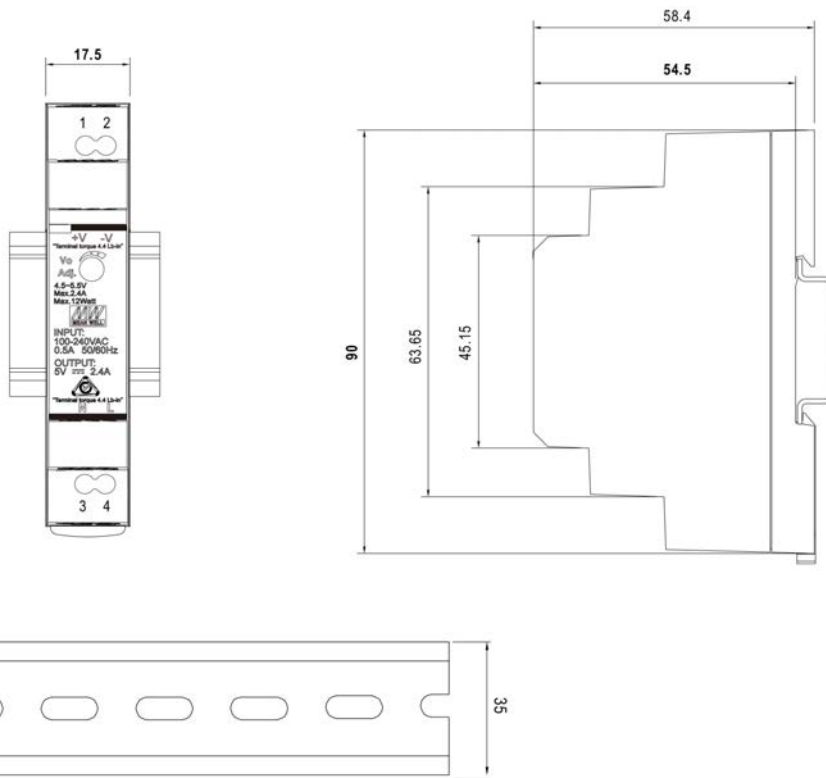
Fig. 2 Abmessungen Netzteil PSU2415
