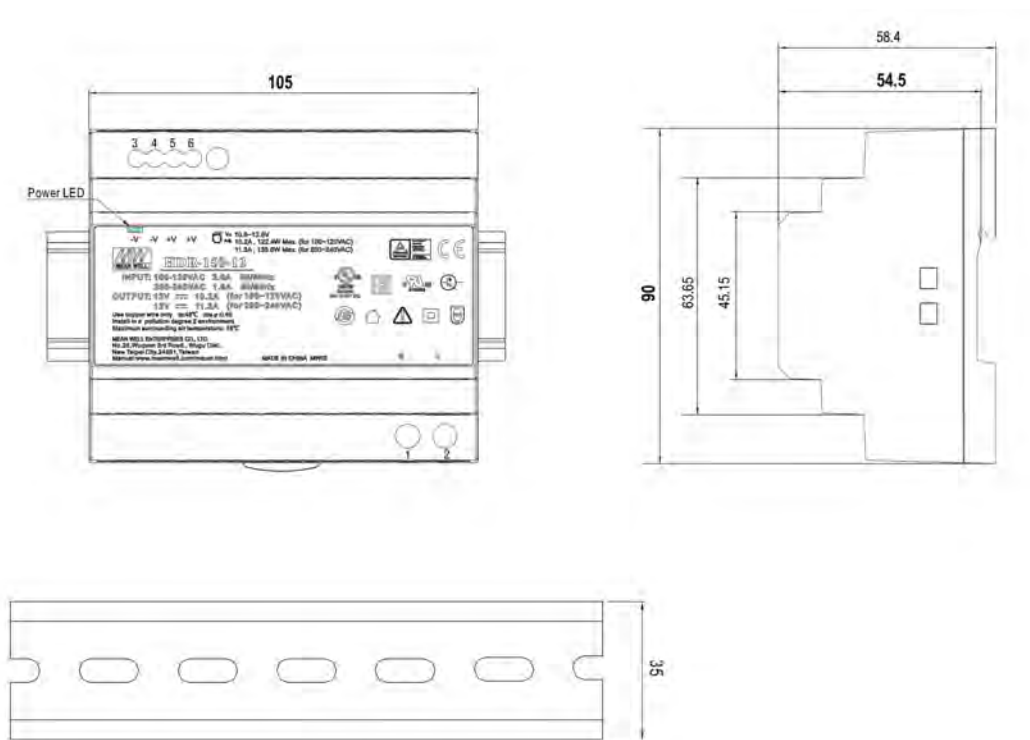
Fig. 2 Dimension bloc d'alimentation PSU24150
