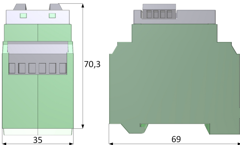
Fig. 1 Dimensions VSM100
