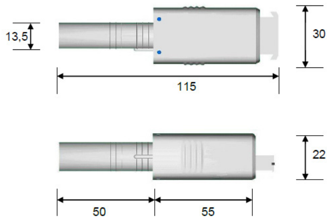
Fig. 2 Maßzeichnung KLC2002
