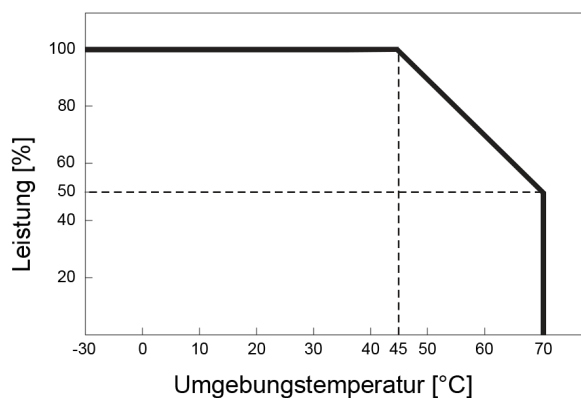
Fig. 3 Leistungsreduktion in Abhängigkeit von der Umgebungstemperatur
