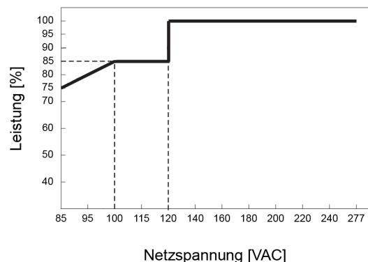
Fig. 4 Leistungsreduktion in Abhängigkeit von der Netzspannung
