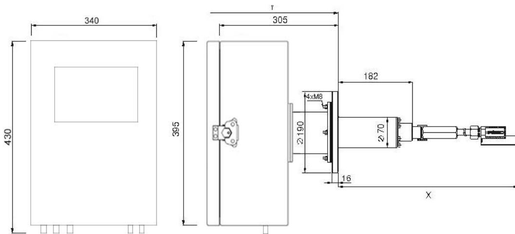
Fig. 1-2 Dimensions
