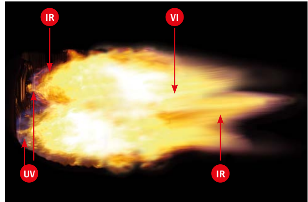
Spektrum der Flamme.
