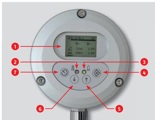
Organe d'affichage et de commande F300K avec UI.
