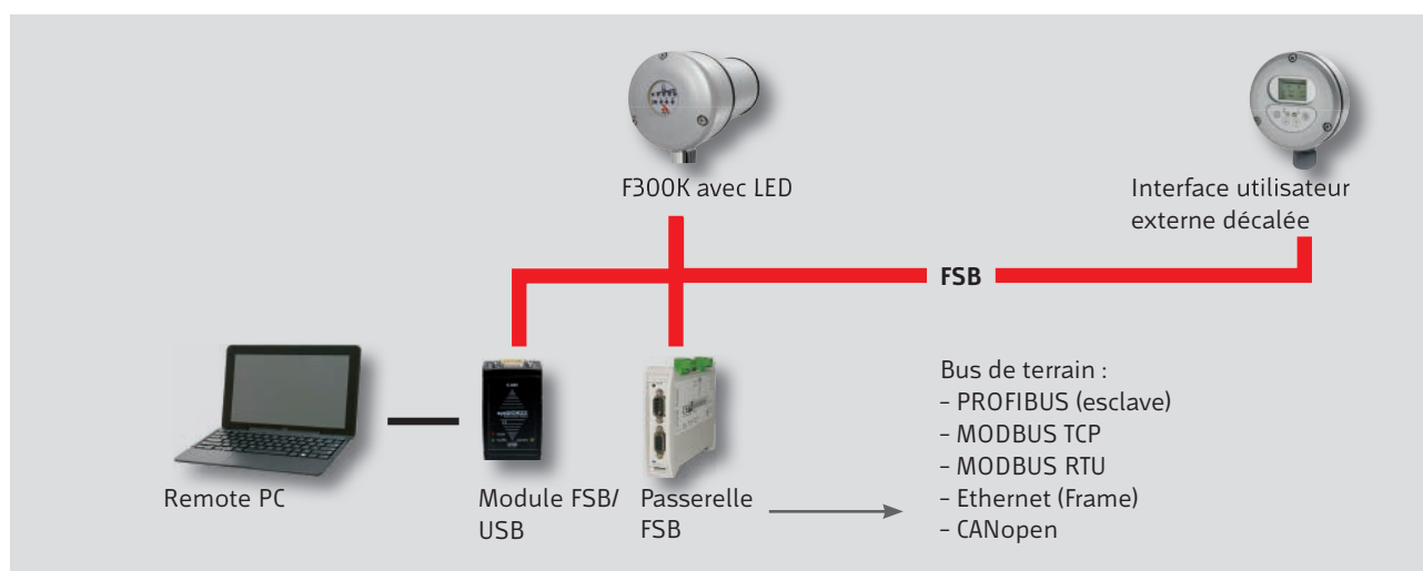
Exemple : Mise en réseau avec un F300K.
