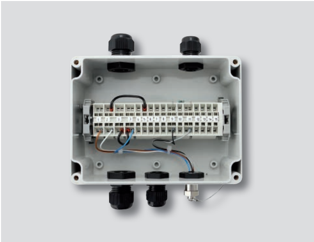
Boîtier FG30-00.
