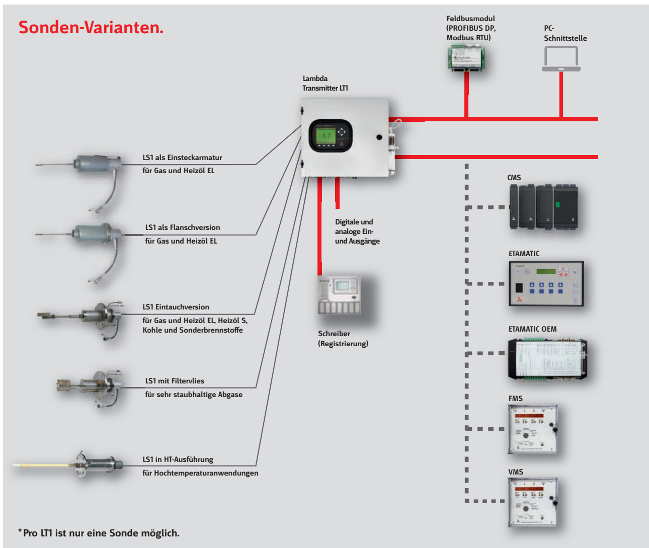
Funktionsübersicht LT1.
