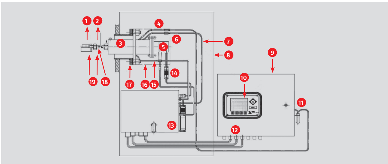
Prinzipieller Aufbau mit externer Messgaspumpe und Abgleicheinrichtung.
