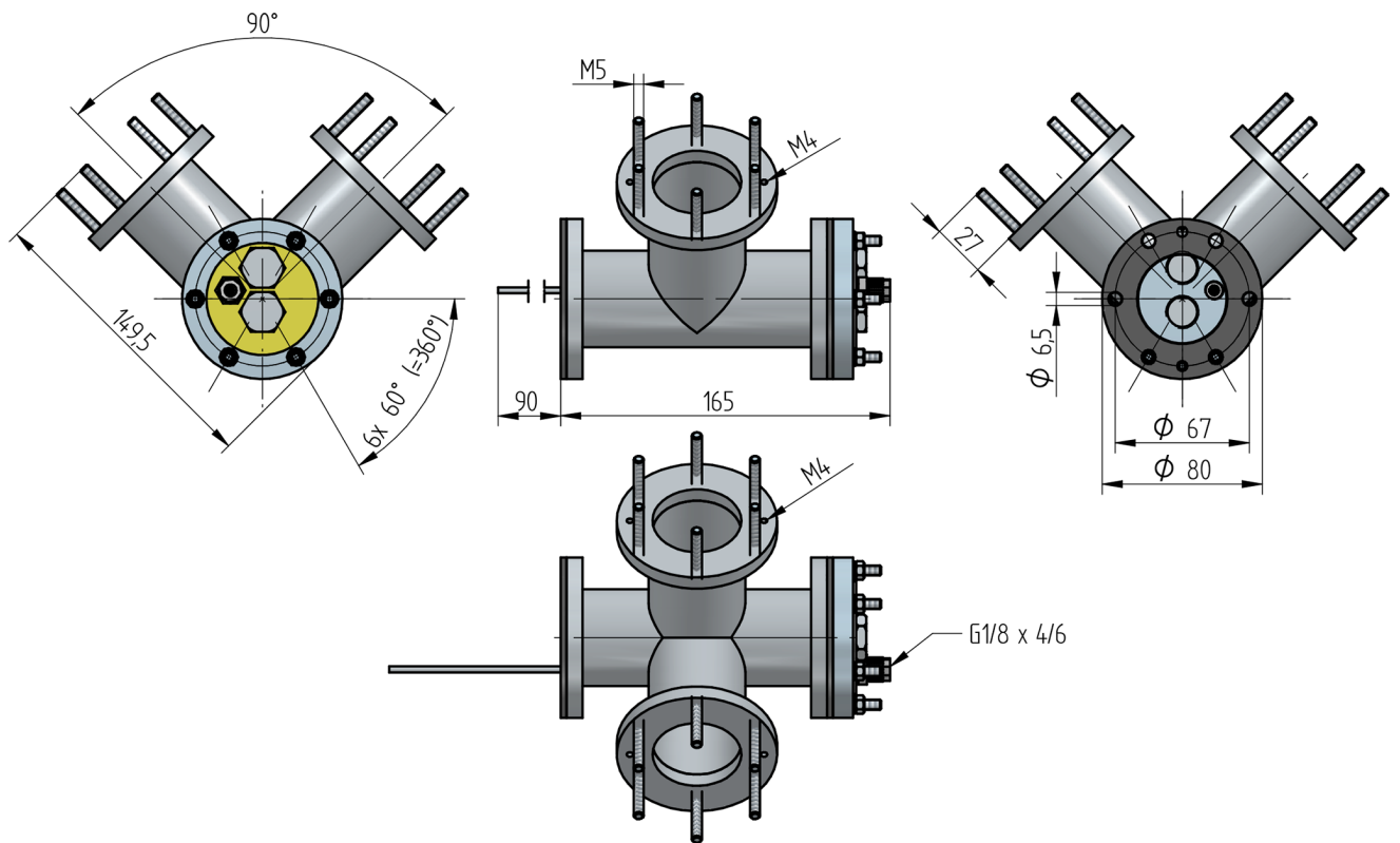
Fig. 1 Adaptateur T pour le logement de sonde pour accélération injecteur
