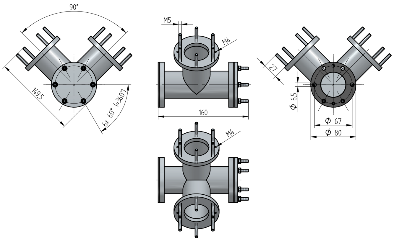
Fig. 1 Adaptateur V standard avec bride aveugle
