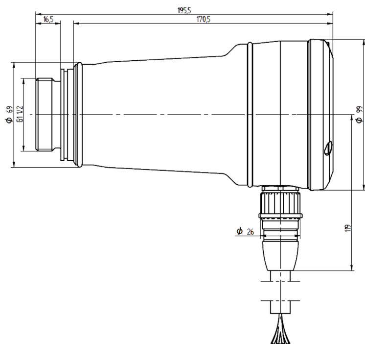
Fig. 3 Plan coté F300K
