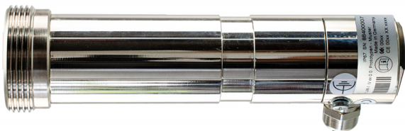
Fig. 1 Détecteur de flamme FFS30 variante à câble
