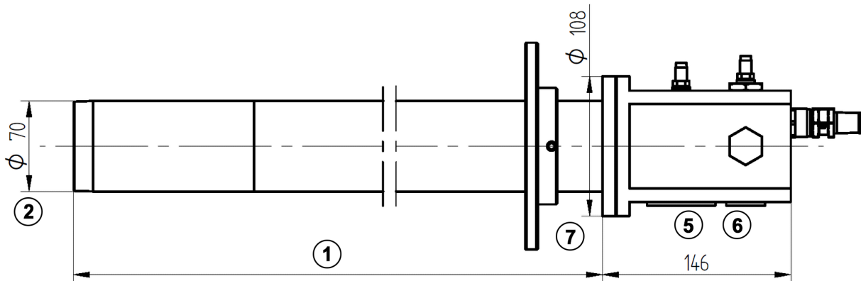
Fig. 4 Dimensions du brûleur d'allumage GFI70 modèle C
