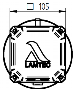
Fig. 5 Vue latérale unité de puissance intégrée zone de sécurité Fig. 6 Dimensions unité de puissance intégrée zone de sécurité
