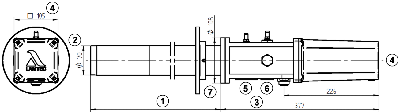
Fig. 2 Dimensions du brûleur d'allumage GFI70 modèles A/B
