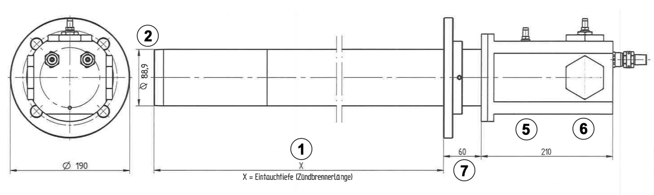
Fig. 6 Dimensions du brûleur d'allumage GF189 modèle C
