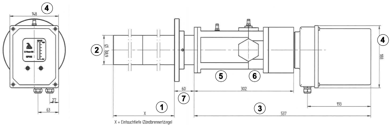
Fig. 2 Dimensions du brûleur d'allumage GF189 modèles A/B
