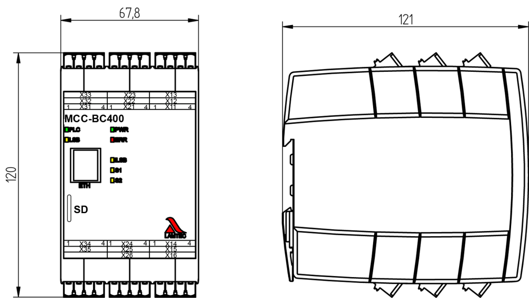
Fig. 2 Plan coté MCC-BC400
