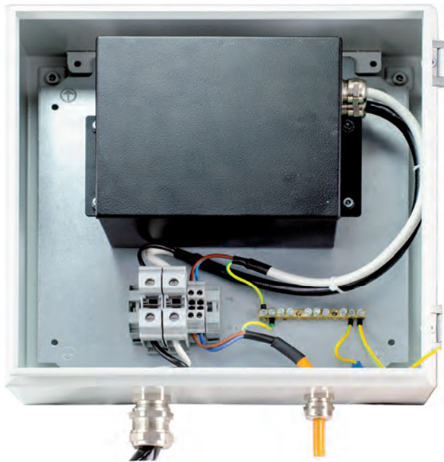
Fig. 1 Externes Stahlgehäuse für Wandmontage Hochenergiezünder HEI500
