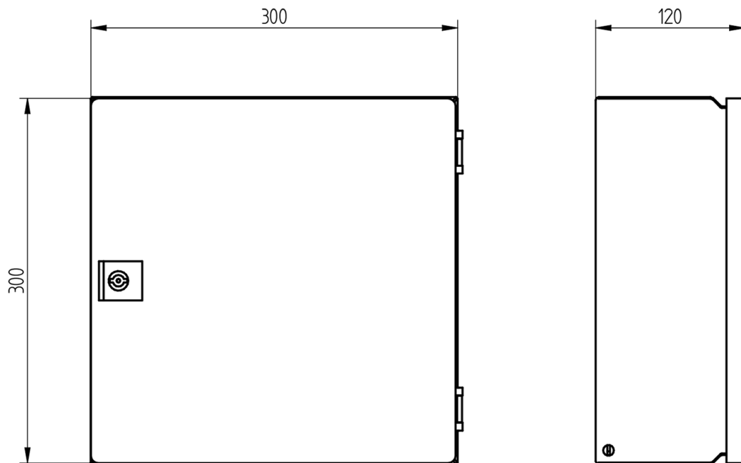
Fig. 2 Abmessungen des externen Stahlgehäuses Hochenergiezünder HEI500
