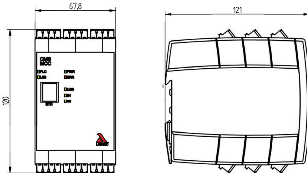
Fig. 2 Maßzeichnung MCC
