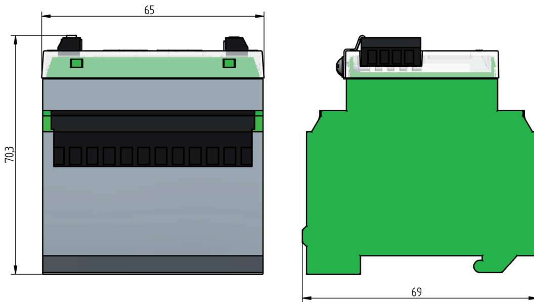
Fig. 1 Abmessungen BT300/EBM102
