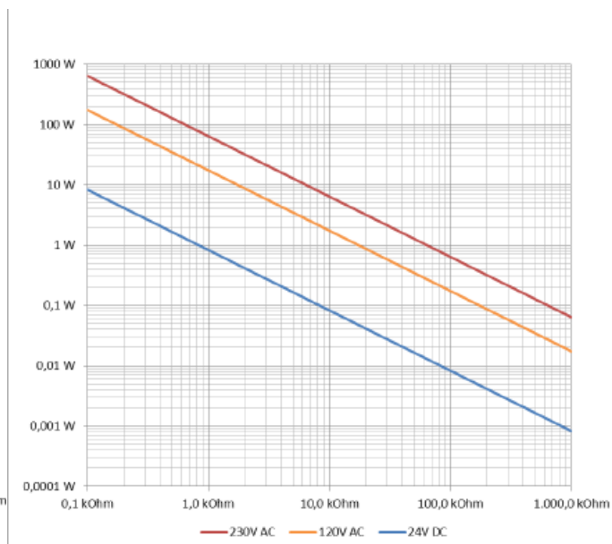
Fig. 5 Puissance de la résistance supplémentaire lorsque la sortie est activée
