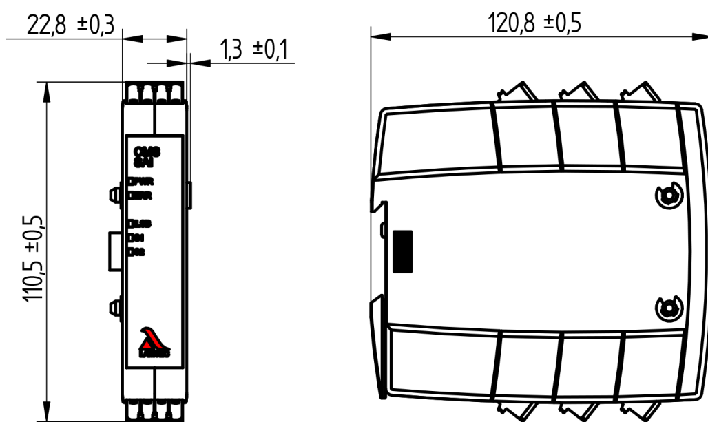
Fig. 2 Dimension SAI
