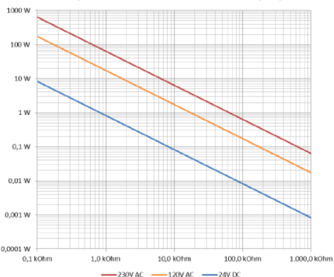
Fig. 5 Leistung des Zusatzwiderstandes bei eingeschaltetem Ausgang
