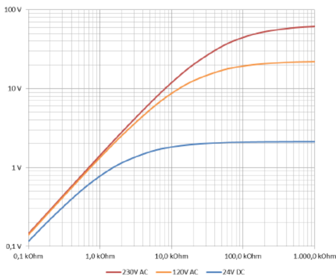
Fig. 4 Restspannung bei ausgeschaltetem Ausgang
