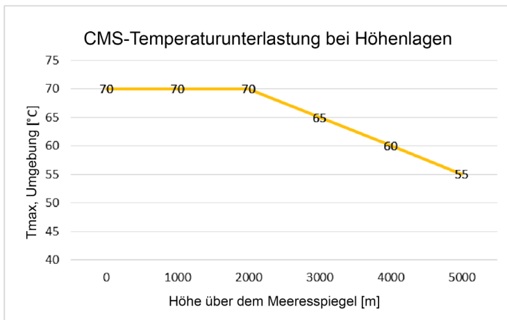
Fig. 3 Temperaturunterlastung für Einsatz >2000m NHN
