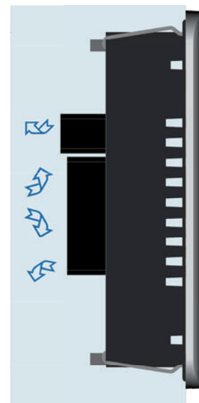
Fig. 2 Freie Luftzirkulation gewährleistet! >20 mm
