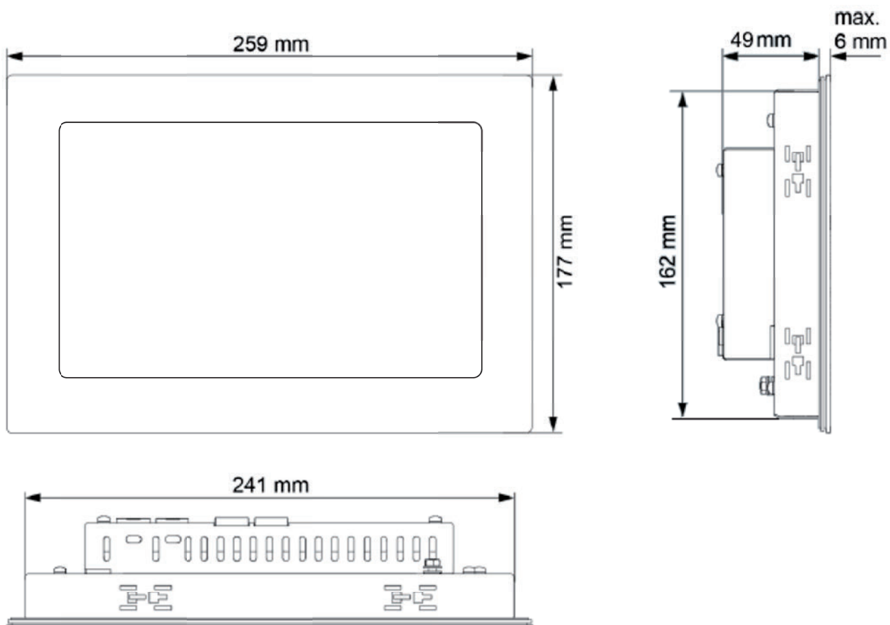
Fig. 3 Maßzeichnung GUI610
