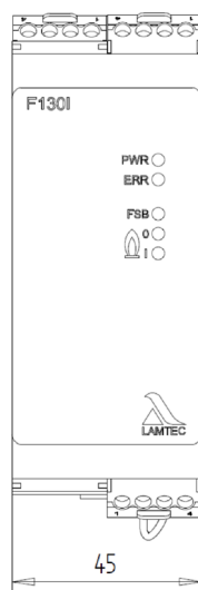
Fig. 2 Dimensions F130I
