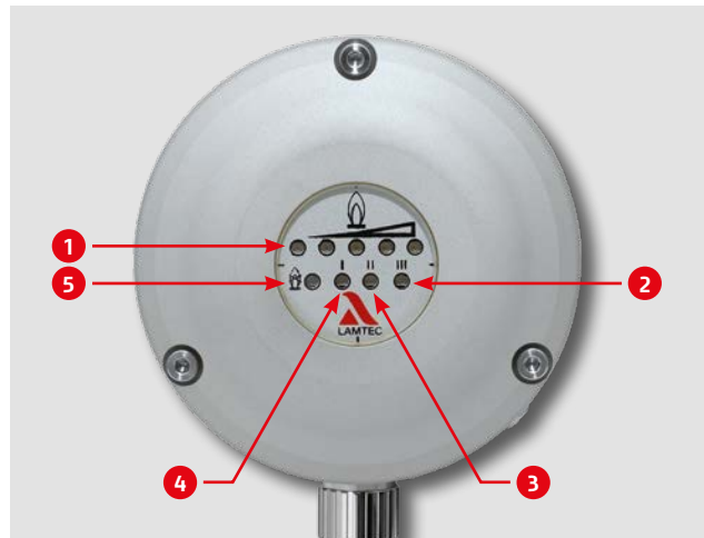
Anzeigeelement F300K mit LED-Anzeige.
