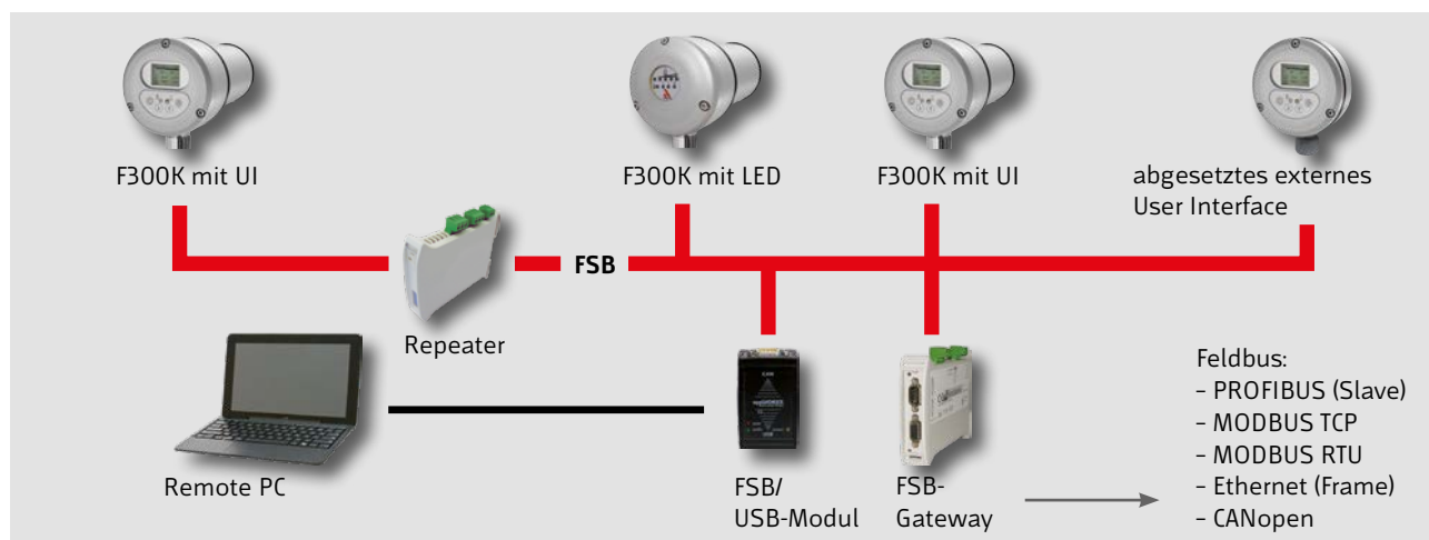
Beispiel: Vernetzung mehrerer F300K.
