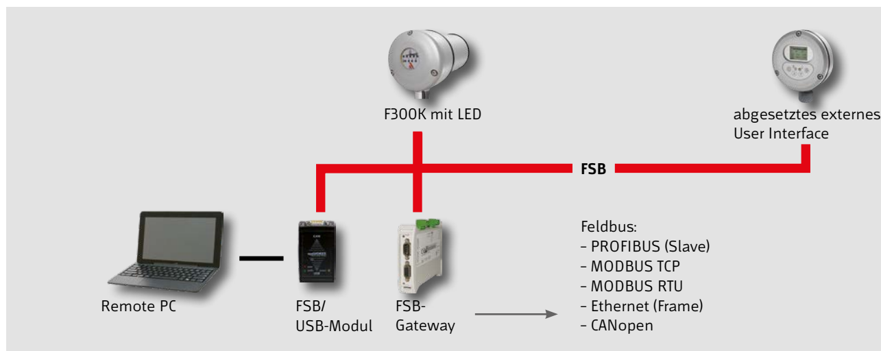
Beispiel: Vernetzung mit einem F300K.
