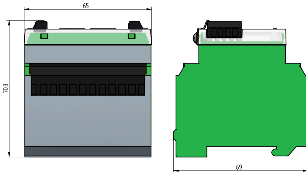
Fig. 1 Abmessungen BC300/EBM312
