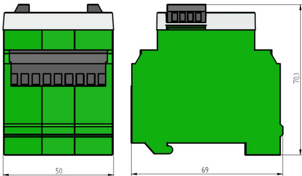
Fig. 1-1 Abmessungen EBM100
