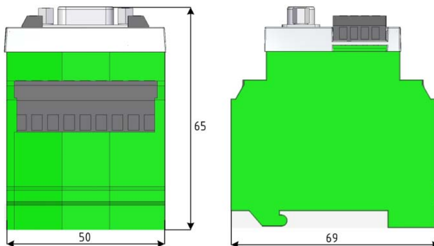
Fig. 1-1 Abmessungen LEM100
