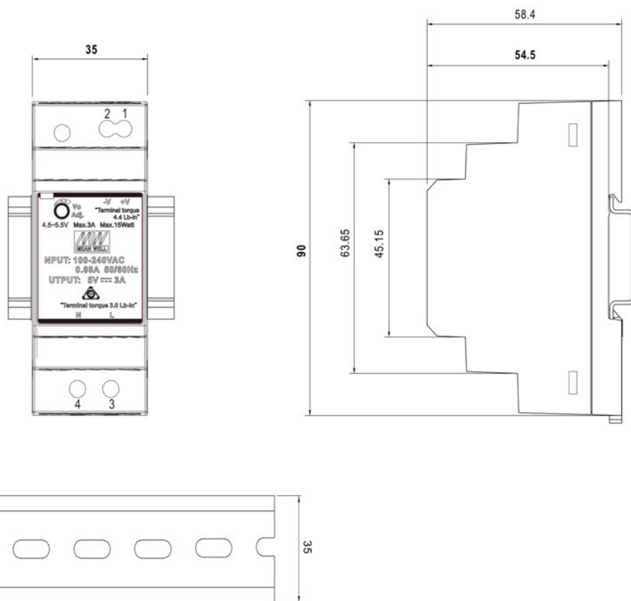
Fig. 2 Dimension bloc d'alimentation PSU2430
