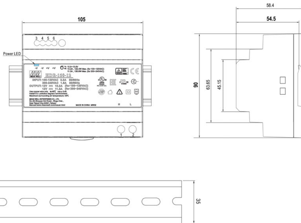
Fig. 2 Dimension bloc d'alimentation PSU24150
