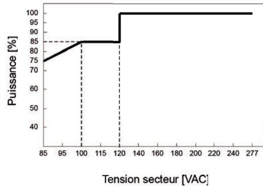
Fig. 4 Réduction de la puissance en fonction de la tension secteur
