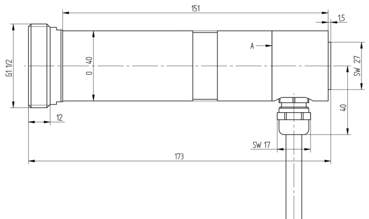
Fig. 4 Maßzeichnung Flammenfühler FFS07 Verschraubungsvariante
