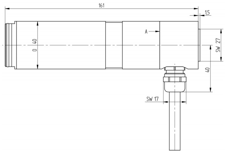
Fig. 2 Maßzeichnung Flammfühler FFS07 Einsteckvariante
