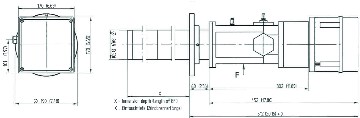
Fig. 4 Abmessungen GFI89 Zündbrenner Ex-Zone 2
