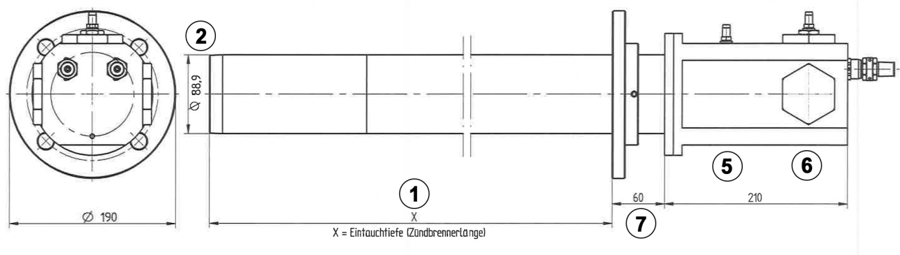
Fig. 6 Abmessungen GFI89 Zndbrenner Ausfhrung C
