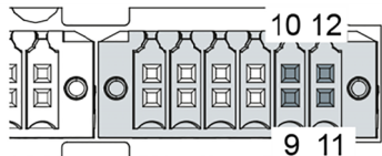
Fig. 6 GUI615 X1 PIN Belegung
