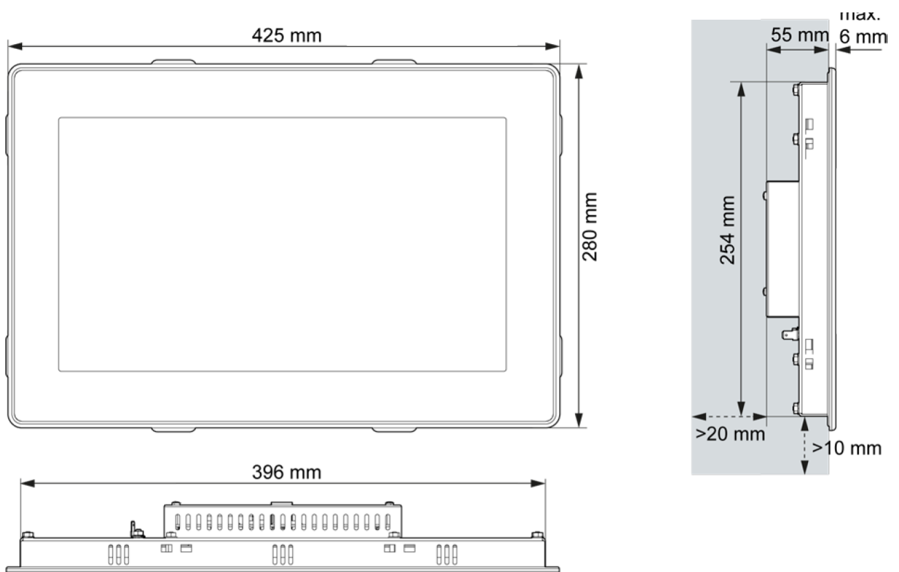
Fig. 3 Maßzeichnung GUI615
