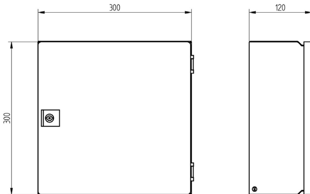
Fig. 2 Maße Gehäuse Hochenergiezündler HEI500
