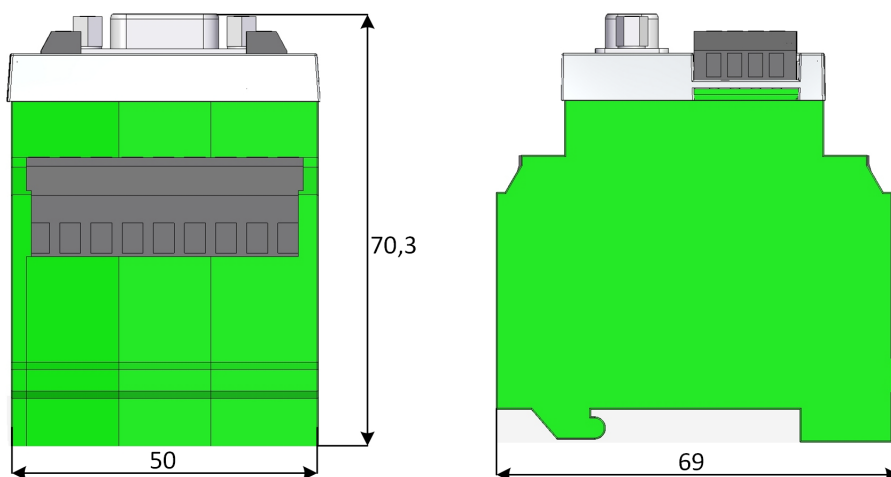
Fig. 1 Abmessungen LEM100
