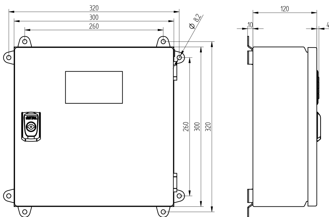
Fig. 3 Maßbild LT3 Gehäuse mit Wandhalterung vertikal/horizontal und UI300-LT-V2 (Maße in mm)
