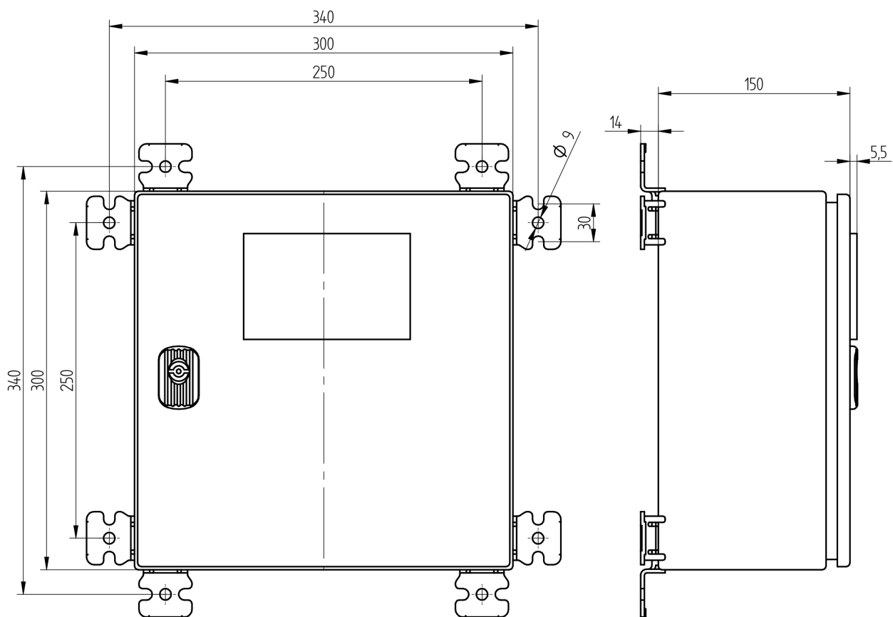
Fig. 4 Maßbild LT3 Edelstahlgehäuse mit Wandhalterung vertikal/horizontal und UI300-LT-V2 mit zusätzlicher Abdeckung für IP65 (Maße in mm)
