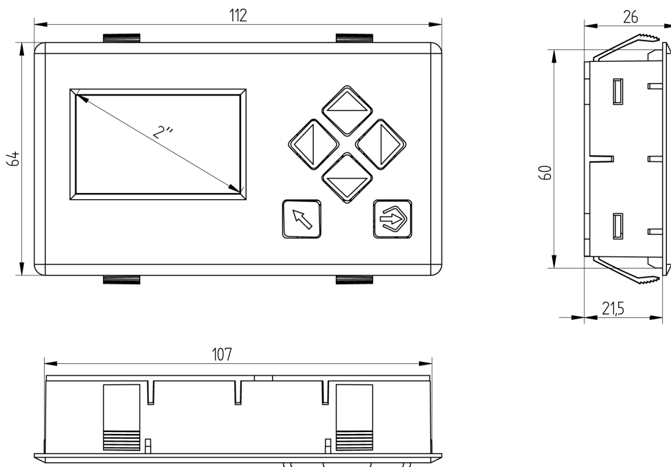
Fig. 2 Maßzeichnung UI300-LSB
