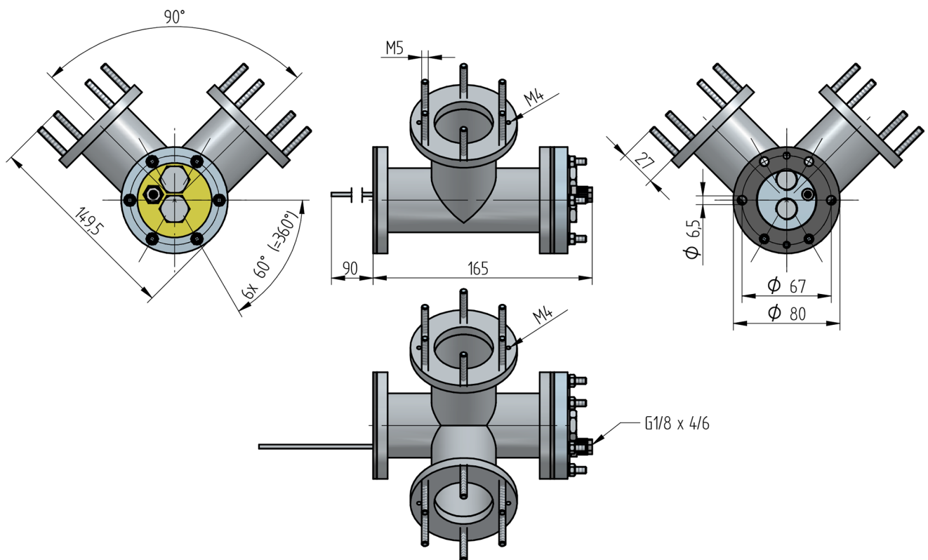
Fig. 1 V-Adapter zur Sondenaufnahme für Injektorbeschleunigung
