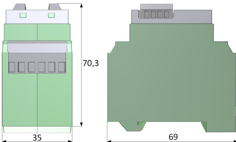
Fig. 1 Abmessungen VSM100
