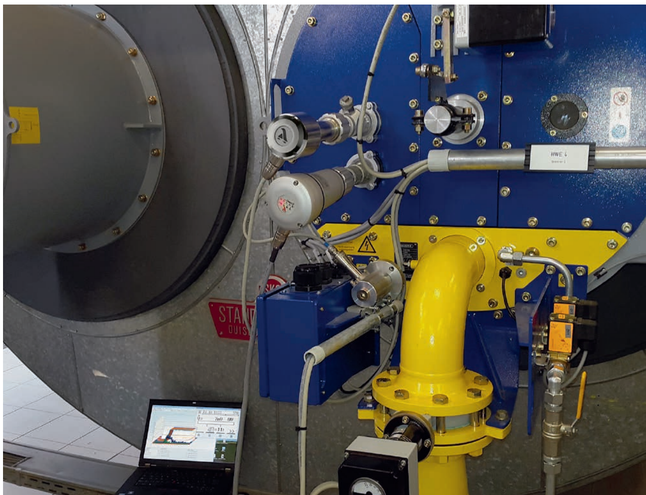
处于工作状态的 LAMTEC火焰监测器F300K
