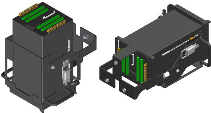
FMS monté dans le support pivotant Type 663R8035 — Position repos (à gauche) position travail (à droite)
