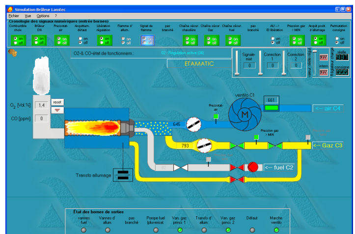
Interface logiciel BSIM
