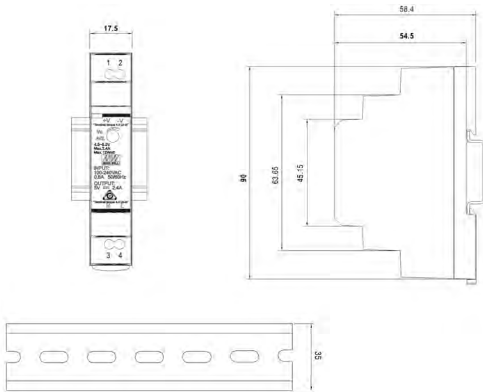
Fig. 2 Dimension bloc d'alimentation PSU2415
