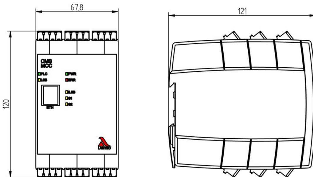
Fig. 2 Maßzeichnung MCC
