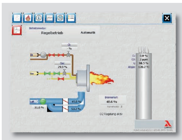
Screenbild Hauptmenü.
