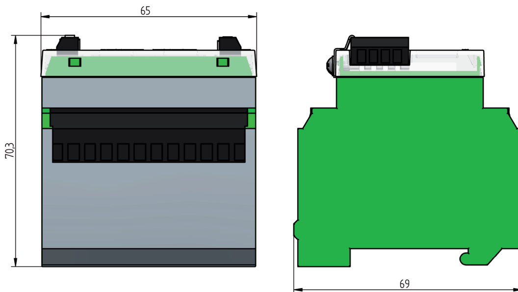
Fig. 1 Dimensions BC300 /EBM312
